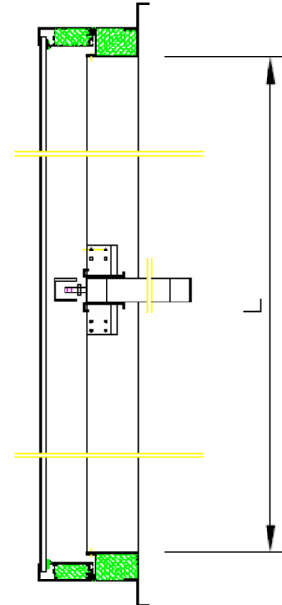
Podélný řez
