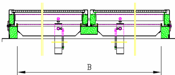
Příčný řez
